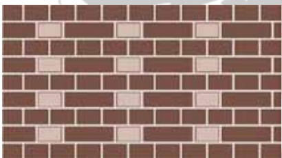
Holländischer Verband
