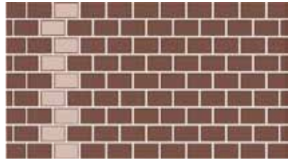
Kopfverband
